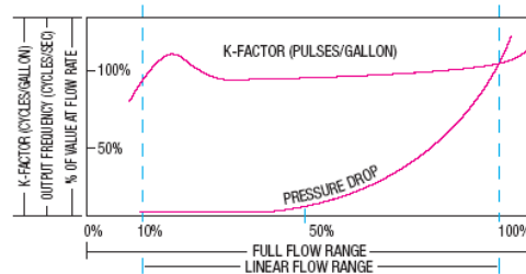
Typical K-Factor Curve (Pulses per Gallon)
